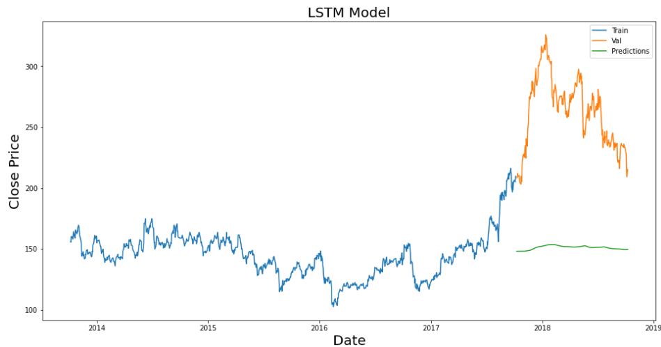
Figure 8. Predicted Value - Actual Value result 3
